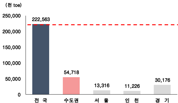
<표 II-34> 최종에너지 소비량
